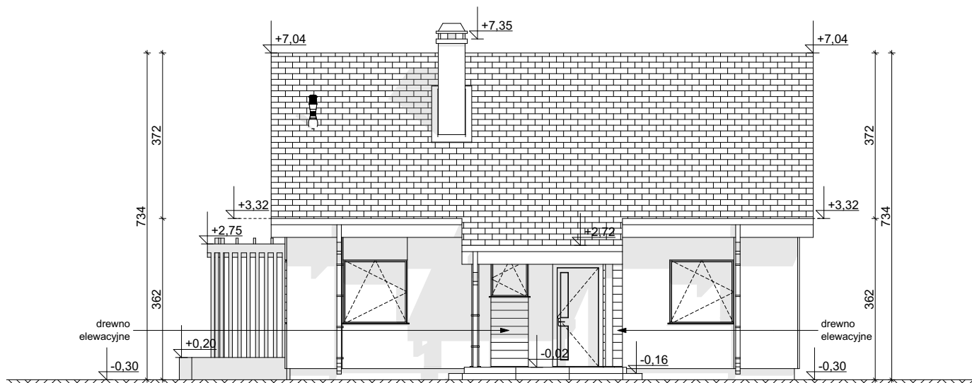
ELEWACJA FRONTOWA
