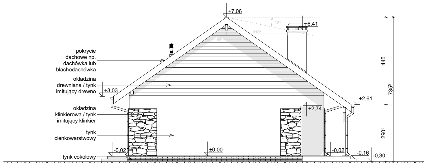
ELEVACJA BOCZNA
