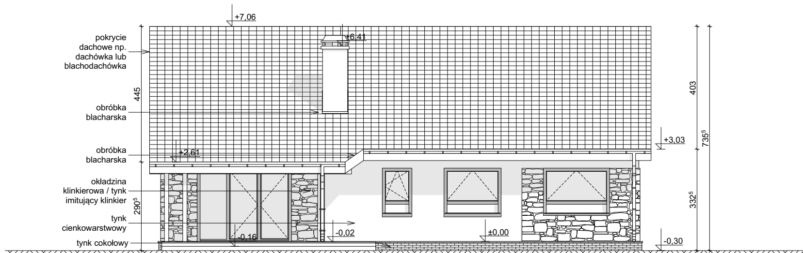
ELEVACJA OGRODOWA
